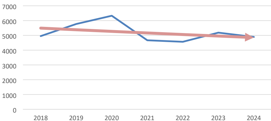
Figur 2: Utvikling påtaleunntatelser etter §70 / Trend i Norge uten Trøndelag
