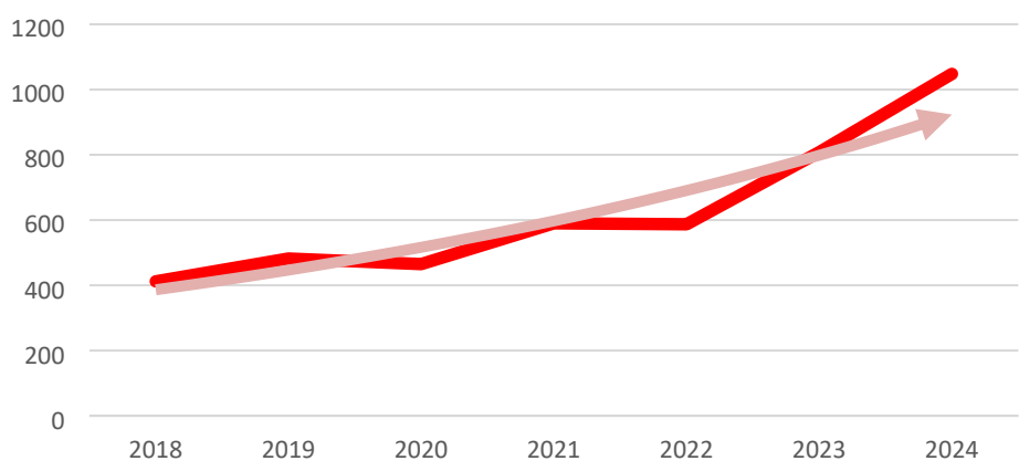
Figur 1: Utvikling påtaleunntatelser etter §70 / Trend i Trøndelag
